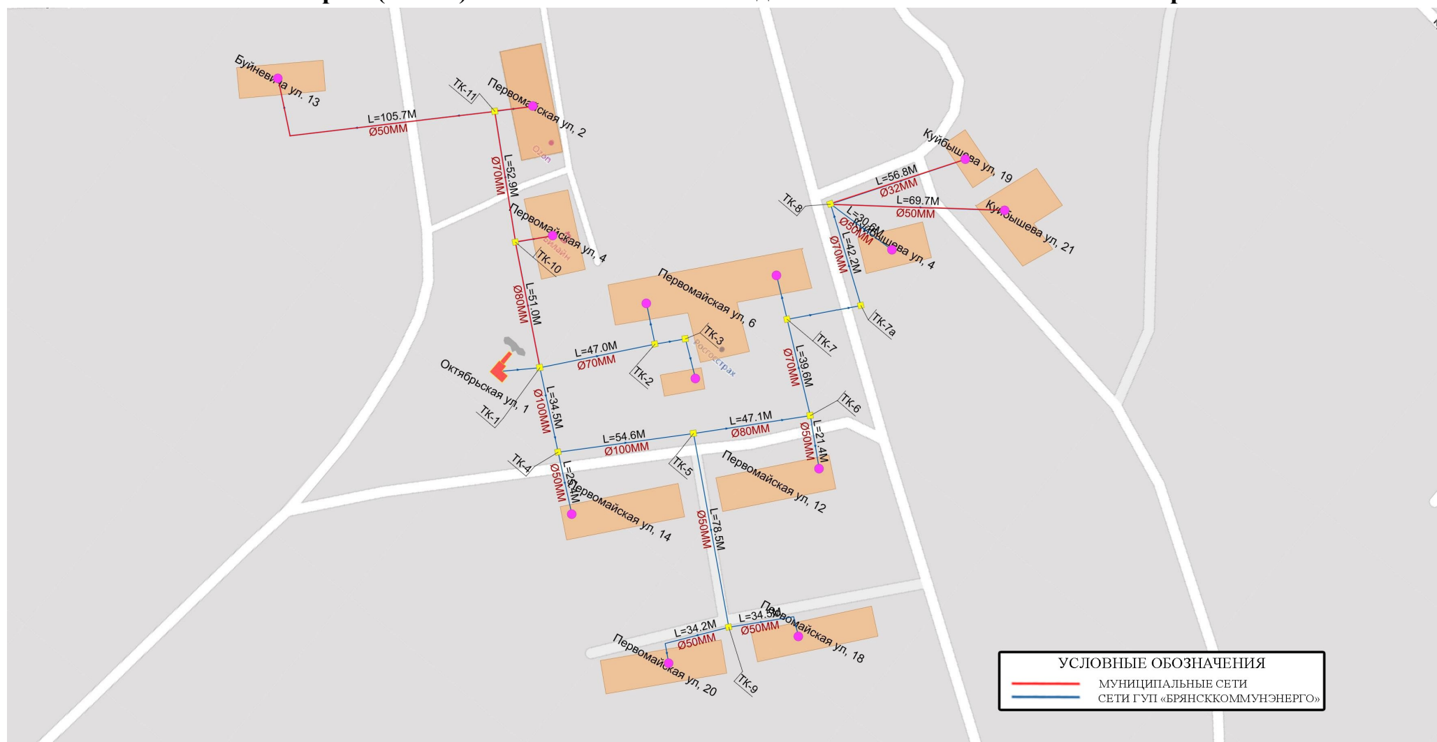
Рис.2.Схема тепловых сетей п. Красная Гора, кот. 1, ул. Октябрьская, 1Б
